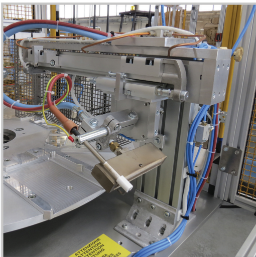
Dispositivo di pre-ffiamatura (accensione automatica e centralina di sicurezza - aria e gas propano) Pre-flaming device (with automatic ignition and gas safety system - air and propane gas)
