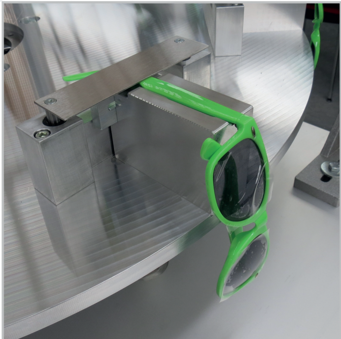
STAZIONE DI CARICO MANUALE MANUAL LOADING STATION
