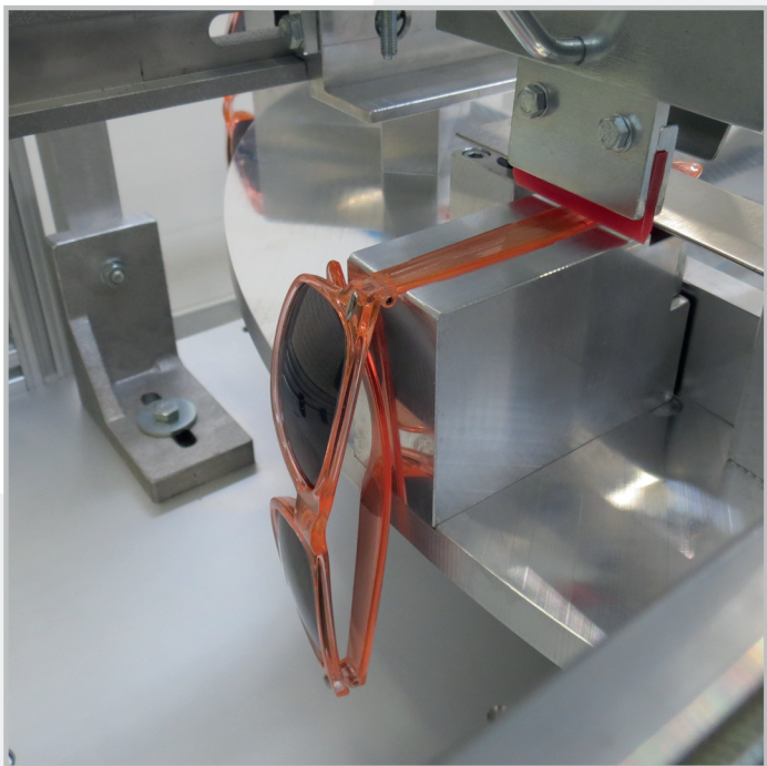
STAZIONE DI STAMPA PRINTING STATION
