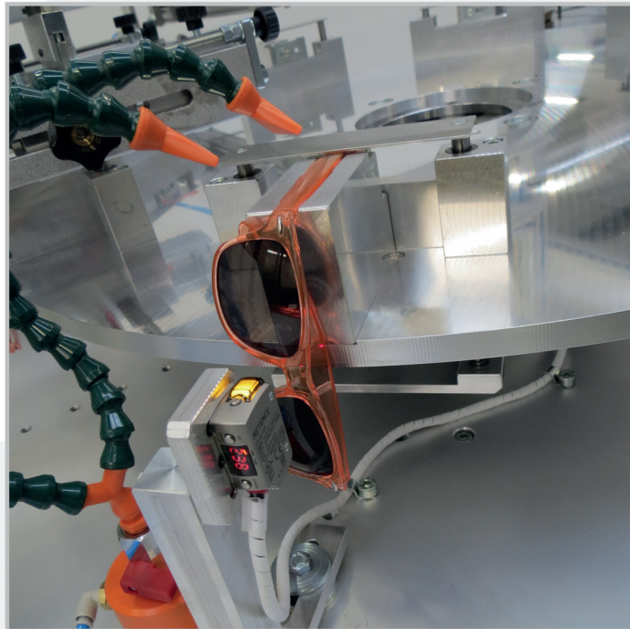
NO OBJECT NO PRINT + SISTEMA DI PULIZIA NO OBJECT NO PRINT + CLEANING DEVICE
