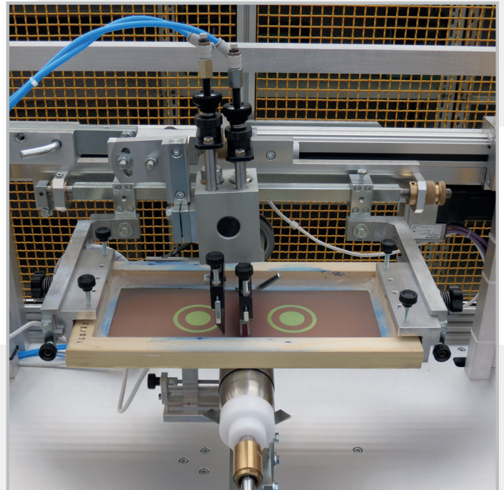
пневматическая система ракеля и электронное перемещение осей PNEUMATIC SQUEEGEE AND ELECTRONIC MOVEMENT OF THE AXES
