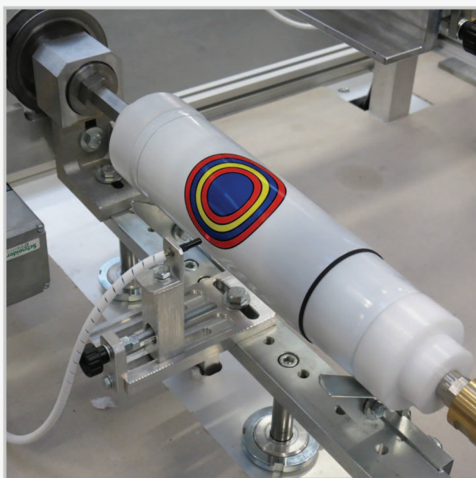
REGOLAZIONE REGISTRO A MEZZO SENSORE E FOTOCELLULA REGISTER ADJUSTING WITH SENSOR AND PHOTOCCELL
