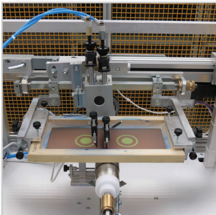
SPATOLA PNEUMATICA E MOVIMENTO ELETTRONICO DEGLI ASSI PNEUMATIC SQUEEGEE AND ELECTRONIC MOVEMENT OF THE AXES
